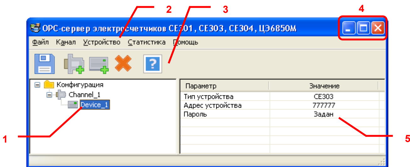
Рисунок 6.1 - Окно конфигурации ОПС-сервера
