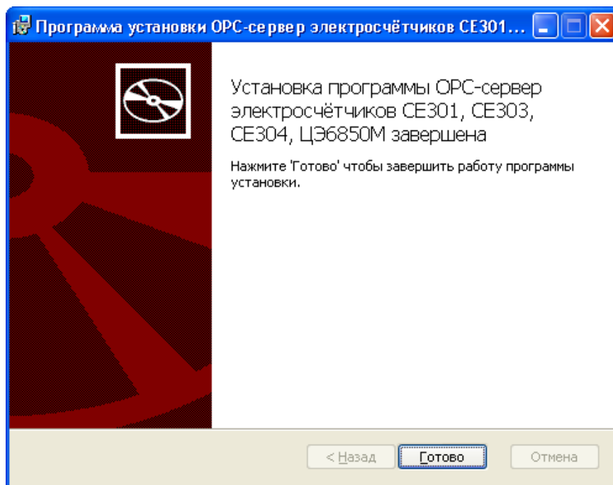
Рисунок 3.5 - Установка завершена
