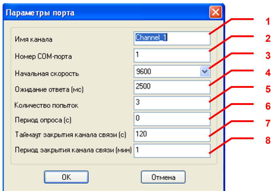
Рисунок 6.4 - Диалоговое окно настройки портов
