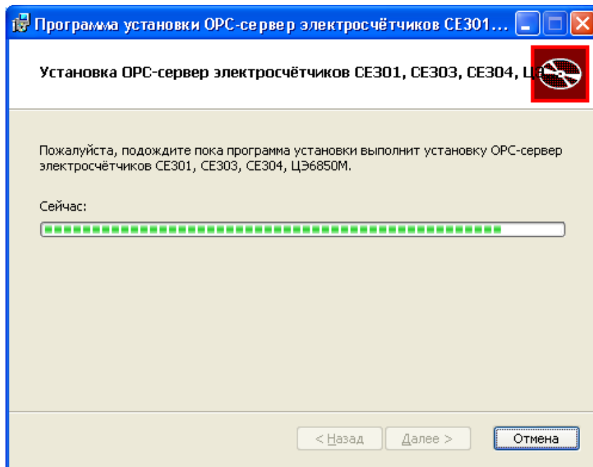
Рисунок 3.4 - Копирование файлов
