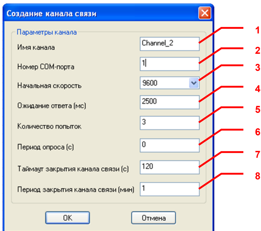
Рисунок 6.3 - Диалоговое окно создания канала связи.
