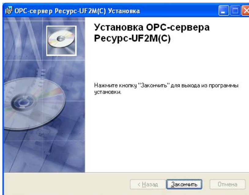
Рисунок 6 - Установка завершена
