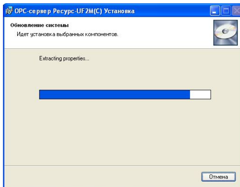
Рисунок 5 - Копирование файлов
